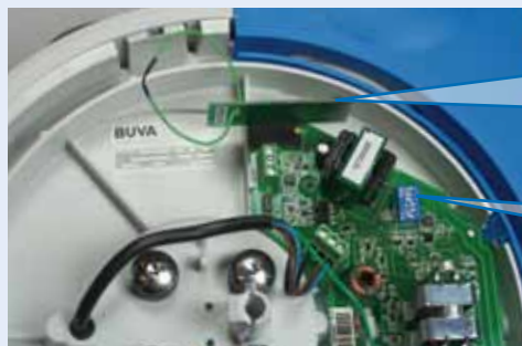
Antenne communicatieprint
