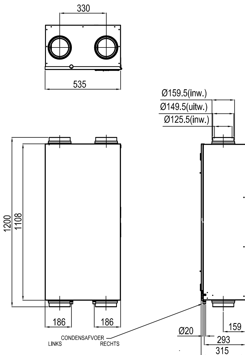
Afbeelding 3.0: Maatschets WHR 920
