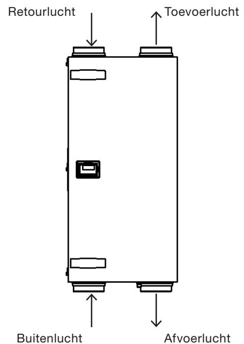
WHR 920 - Rechts
